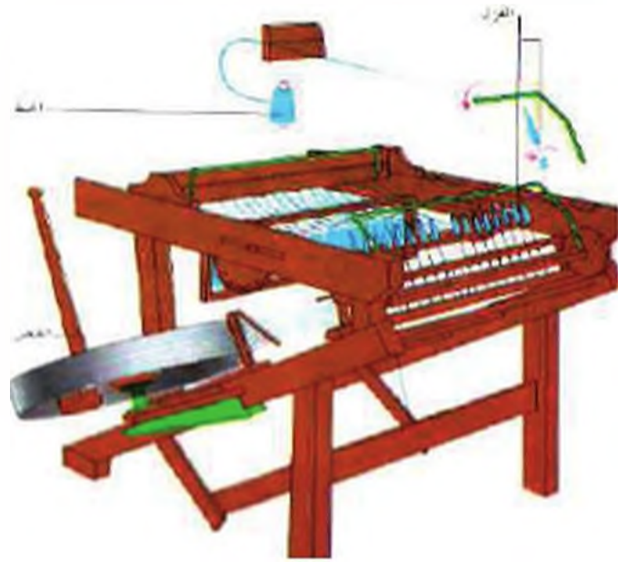
الشكل (٧) مغلز هارجريلز
