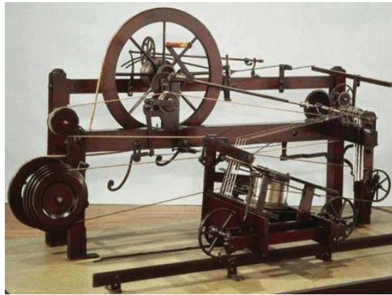
«Ջեննի» ճախարակ
