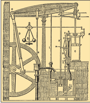
Առաջին շոգեմեքենայի գծագիրը
