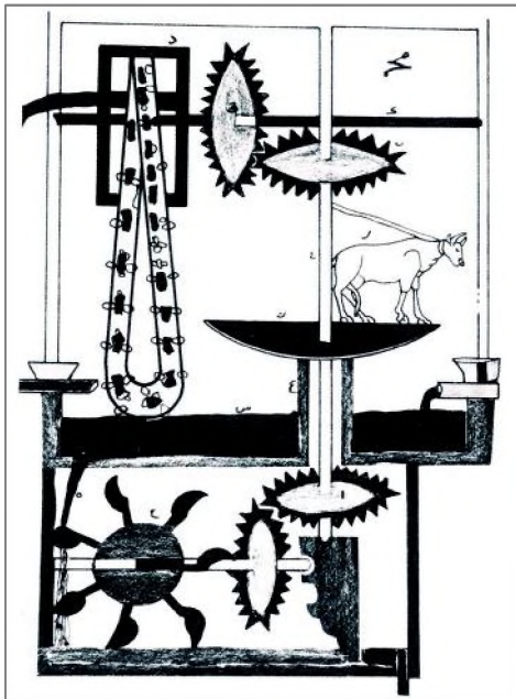
شكل (٤) مخطط مضخة مياه
