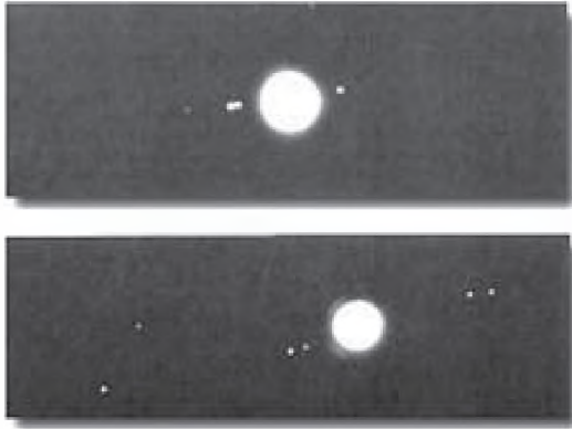
Jupiter et quatre de ses satellites, tels qu'à dû les voir Gallée ...
