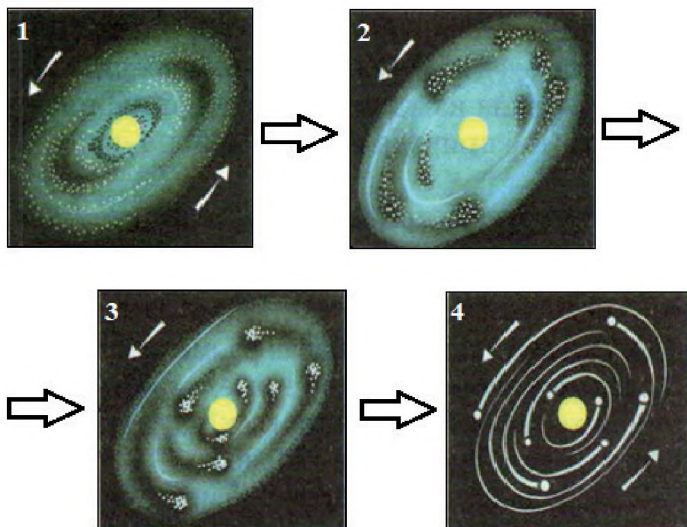
Пайдоиши Манзумаи Офтоб аз абрҳои газу чангӣ
