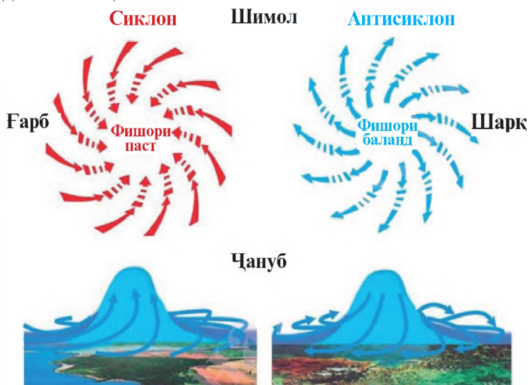
Нақшаи ҳаракати анбӯҳҳои ҳаво дар сиклон ва антисиклон (барои Нимкураи шимолӣ)
