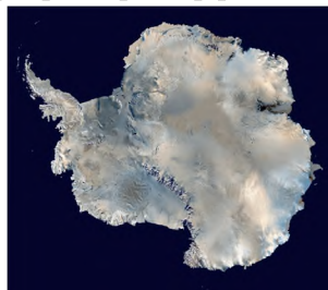
Қабати яхи Антарктида (намуд аз кайҳон)
