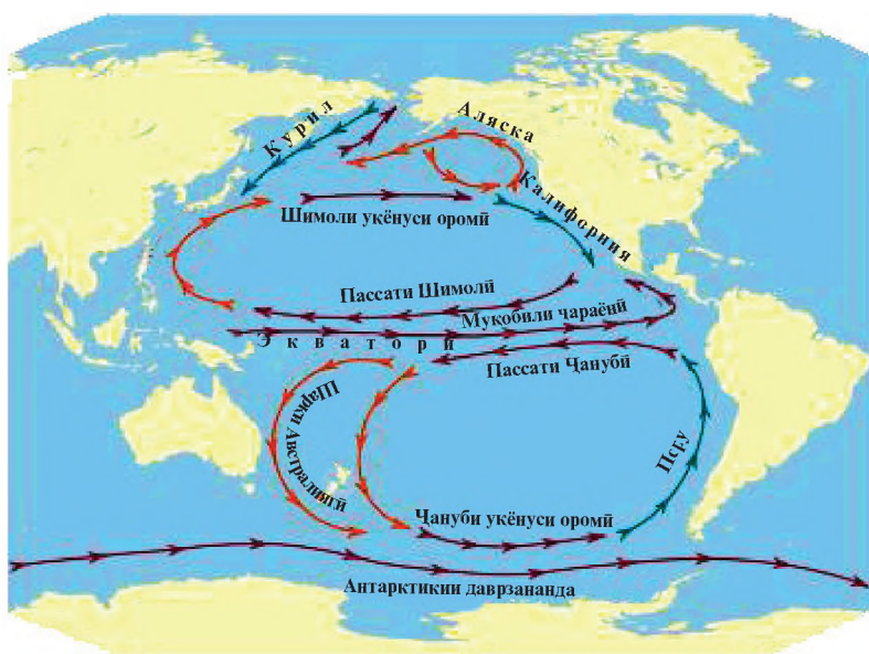
Чараёнҳо дар уқёнуси Ором
