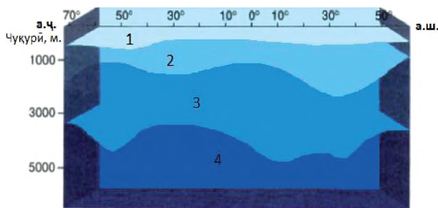
Анбуҳҳои оби уқёуси Атлантик (аз рӯи буриши меридианӣ - аз 70° а.ч. то 60° а.ш.): 1 – сатҳӣ; 2 – мобайнӣ; 3 – чуқуроба; 4 – қаъри
