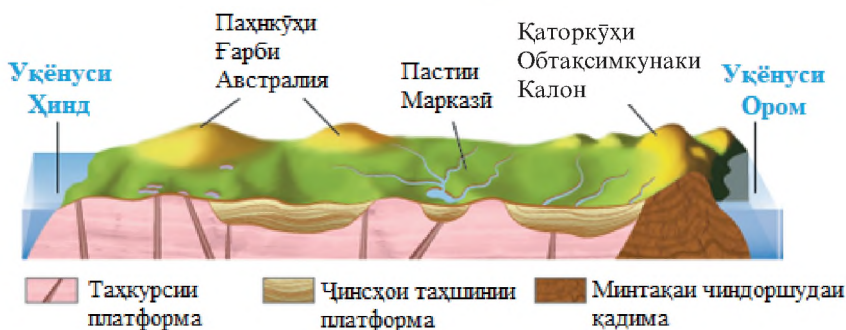
Сохти қири замин ва релефи Австралия (30° а.ҷ.)
