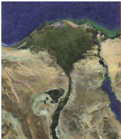
Делтаи дарёи Нил
