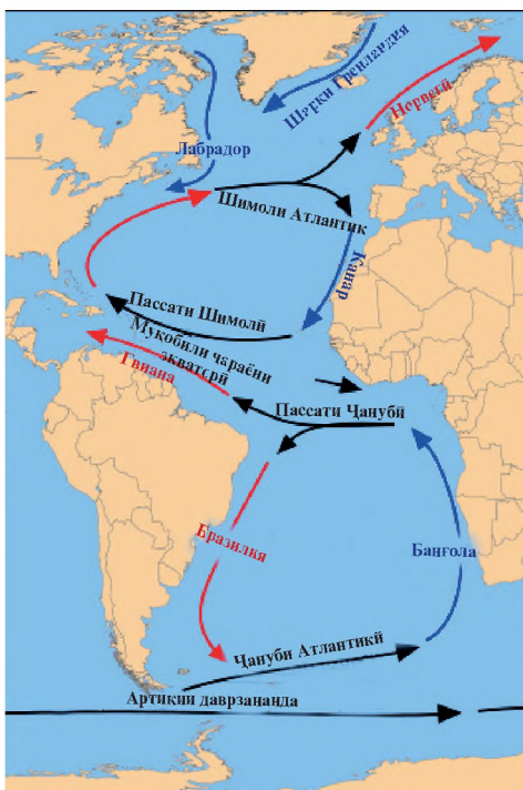
Ҷараёнҳои уқёнуси Атлантик
