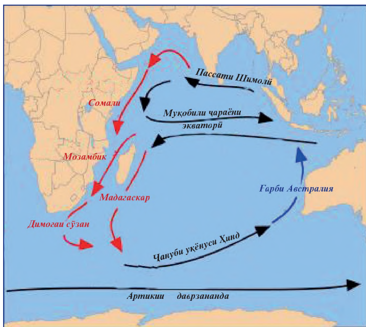
Ҷараёнҳои уқёнуи Ҳинд
