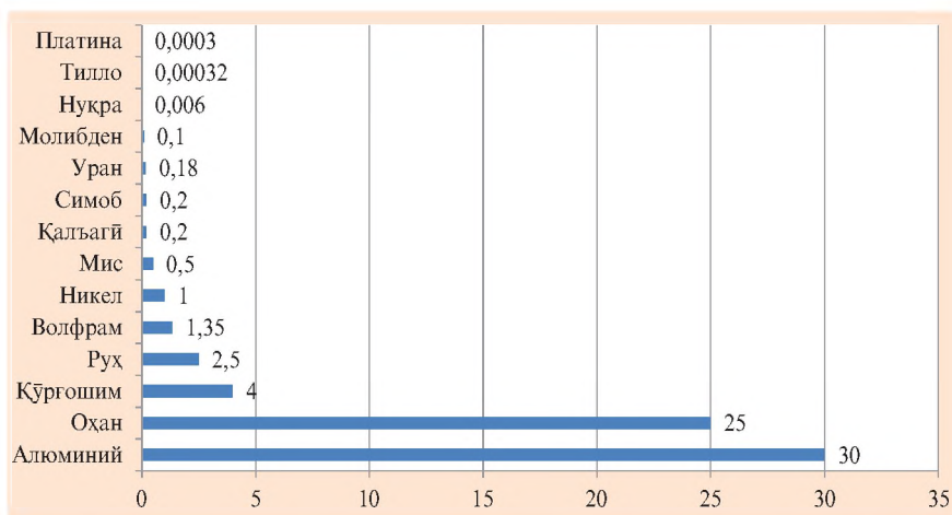
Расми 8. Ҳаҷми минималии мавҷудияти металлҳо дар таркиби маъдан, ки истифодаи онҳо самаранок мебошад.
