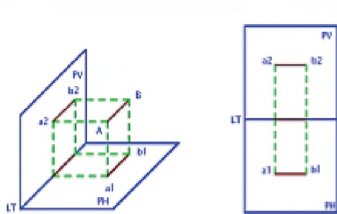
Imagen 6: PROYECCIÓN DIÉDRICA ORTOGONAL DE UN SEGMENTO HORIZONTAL Y SU REBATIMIENTO
