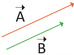
Vectores paralelos
