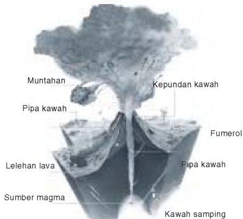
Gambar 1.20 Bagian-bagian dari gunung api
