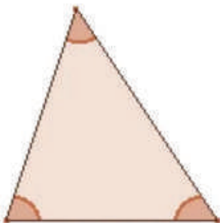
Triángulo Acutángulo
