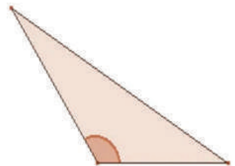
Triángulo Oblicuángulo
