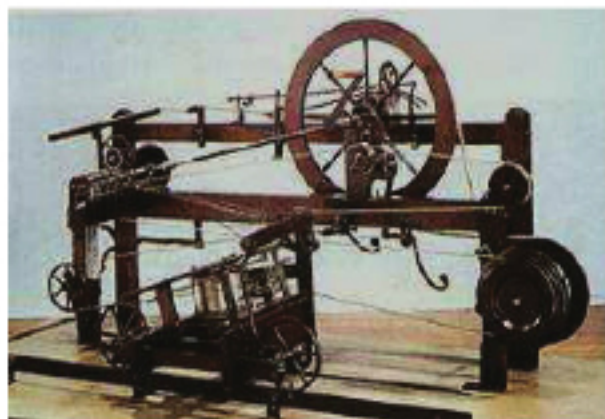
الشكل (٥) اخترع صموئيل كرومبتون المغزل الآلي عام ١٧٧٦م، واستخدمه في غزل القطن.
