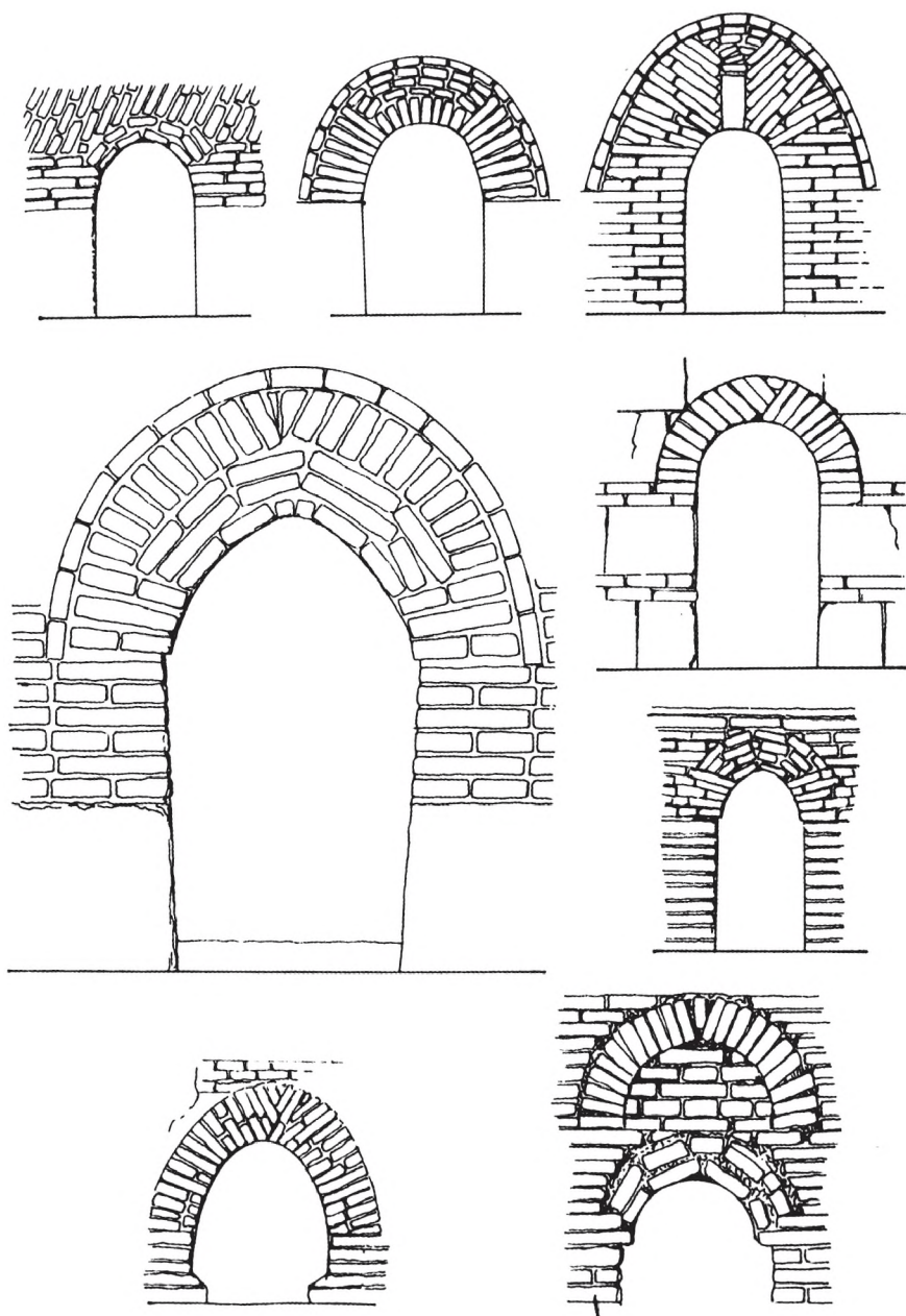
Рисунки 24. Намудҳои арк дар биноҳои асрҳои III–VIII м
