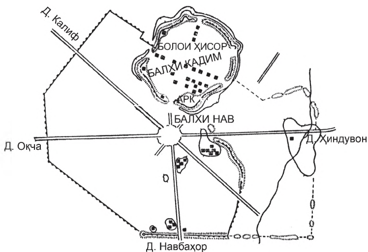
Расми 13. Нақшаи топографии Балх
