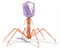
Bacteriofago
