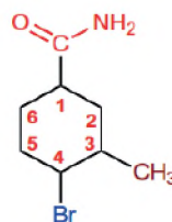
4-Bromo-3-metilciclohexano carboxamida
