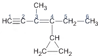
4-ciclopropil-3-metilhexa-3-eno-1-ino
