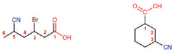
Ácido 3-Bromo-5-cianohexanoico
