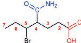
Ácido 5-Bromo-4-carbamoilheptanoico
