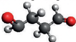
Nomenclatura
