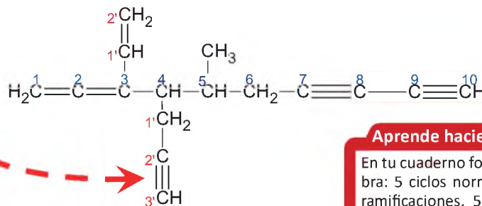
3 - (1'- etenil) - 5 - metil - 4 - (2'- propinil) nona - 1,2- dien - 7,9 - diino
