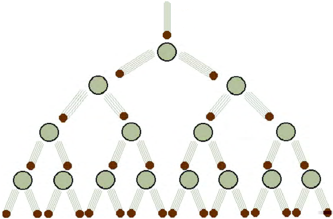
Atomun parçacıklara ayrılmasını gösteren şema.
