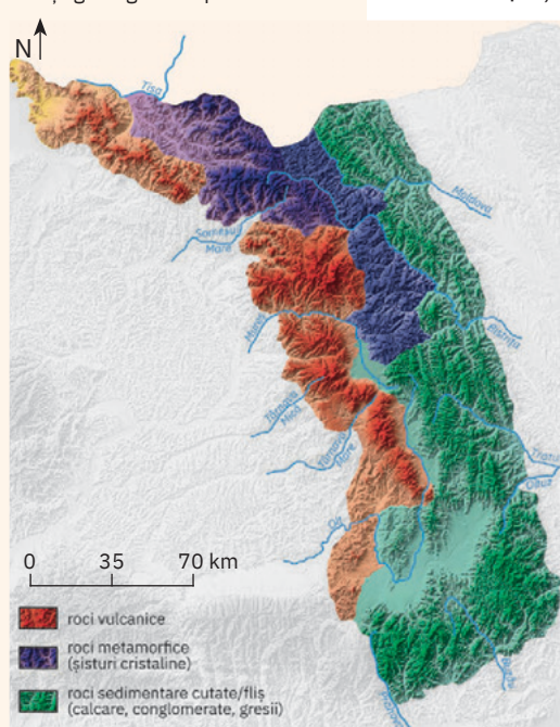
Carpați Orientali. Schiță geologică simplificată
