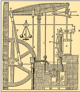
Առաջին շոգեմեքենայի գծագիրը
