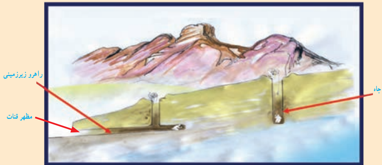
شکل ۳۰-۱- نیم‌رخ از ساختمان یک قنات به‌عنوان یکی از سازه‌های عجیب جهان
