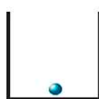
Condensado de Bose - Einstein
