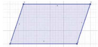
Dado
