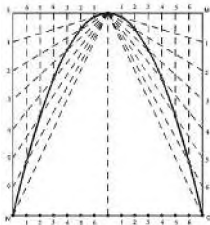
Construcción de la parábola por haces proyectivos
