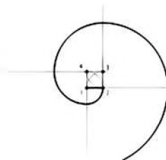
Espiral de cuatro centros
