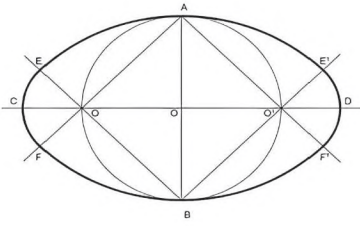
Trazado del Óvalo conociendo el Eje menor
