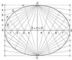
Construcción de la elipse por haces proyectivos
