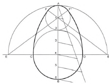
Trazado del Ovoide conociendo el eje mayor
