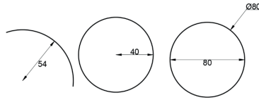
Figura 12. Acotación de arcos, radios y diámetros.
