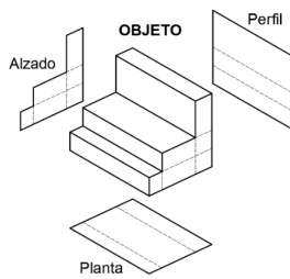
Figura 6. Vistas diédricas (planta, alzado y perfil).
