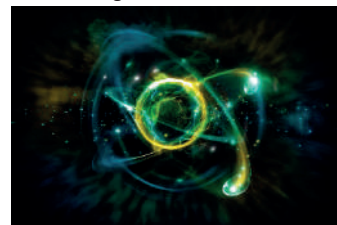
Figura 1: El átomo.
