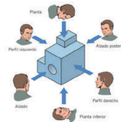
Figura 7. Todas las vistas diédricas.
