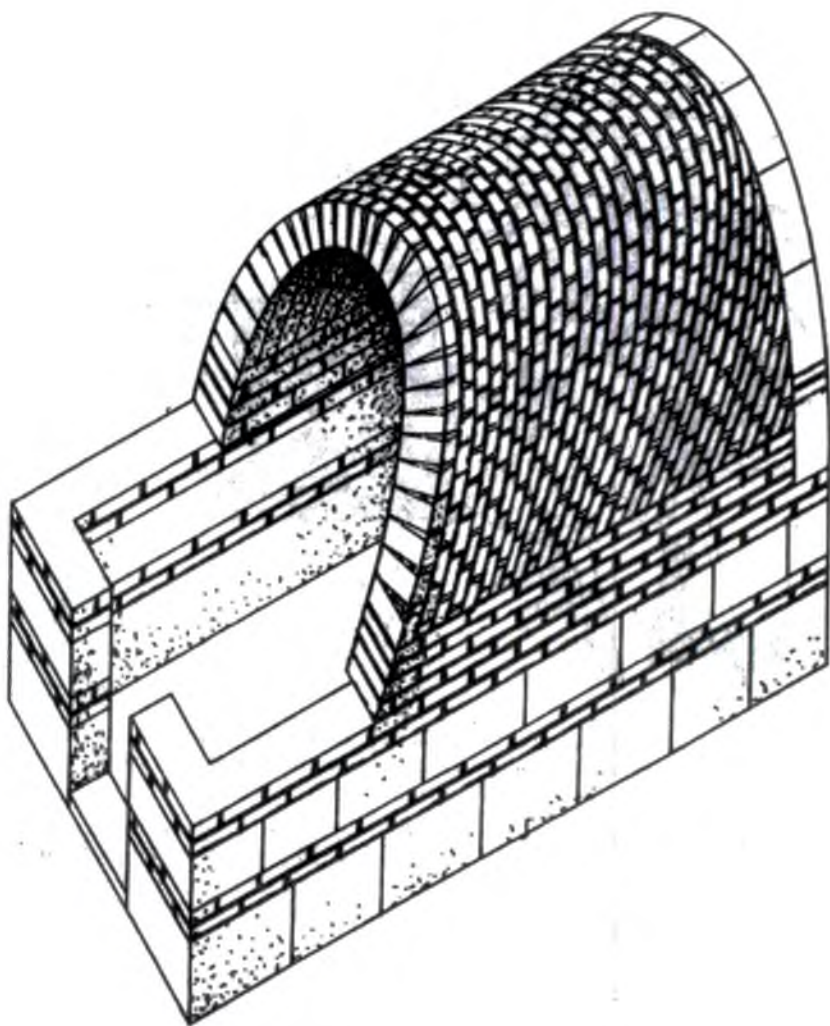
Расми 31. Намуди пӯшиши нимдавра ё равоқӣ.
