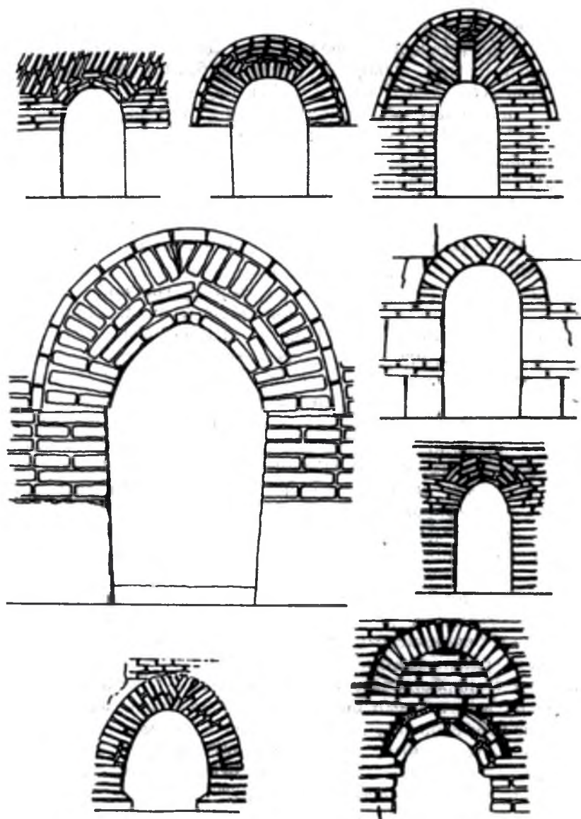
Расми 30. Намудҳои арк дар сохтмонҳои асрҳои III-VIII м.
