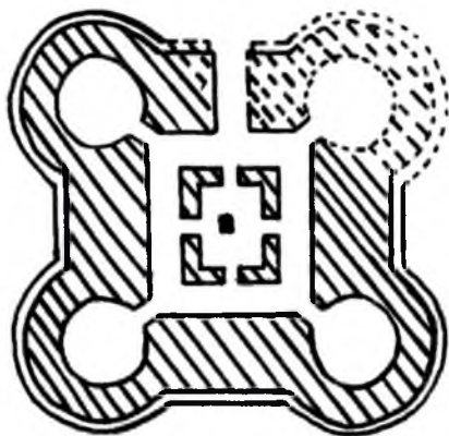
Расми 39. Маъбаи оташ дар ёдгории Октеппа аз чониби бостоншинос А. Пулодов ҳафриёт шудааст.
