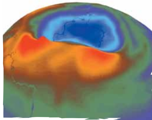
Imagen digital que representa el agujero de la capa de ozono de la zona antártica.
