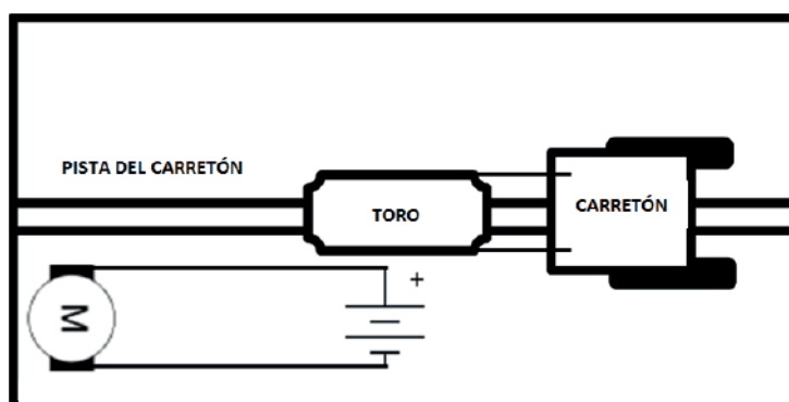
Figura 1. Gráfico de la instalación mecánica y eléctrica del carretón.
